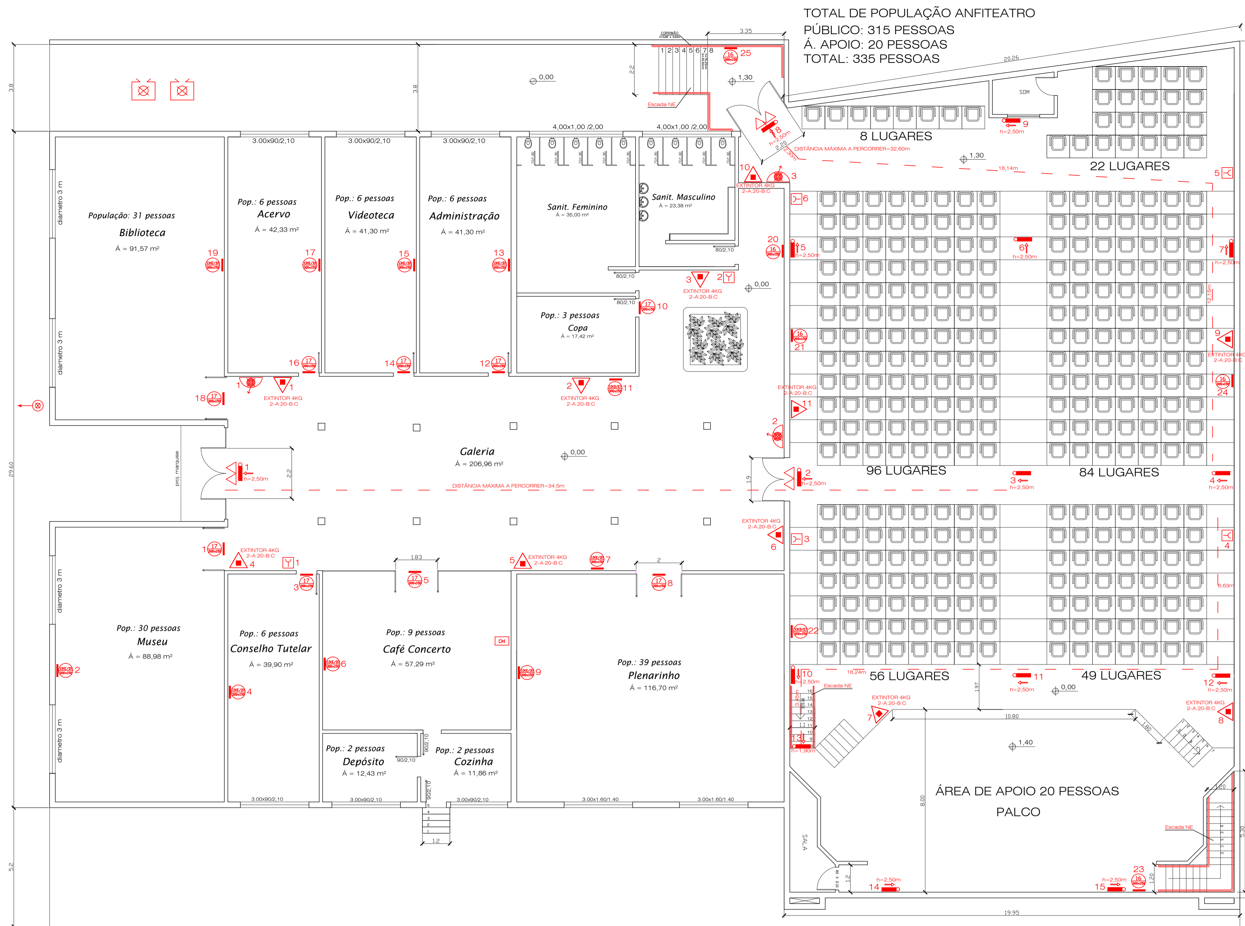
PLANTA BAIXA TÉRREO ÁREA=1625,86m 2 ESCALA 1:100
