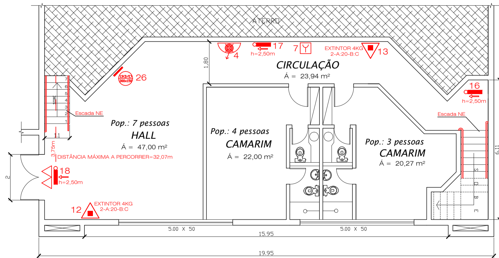
PLANTA BAIXA SUBSOLO ÁREA=150,32m 2 ESCALA 1:100
