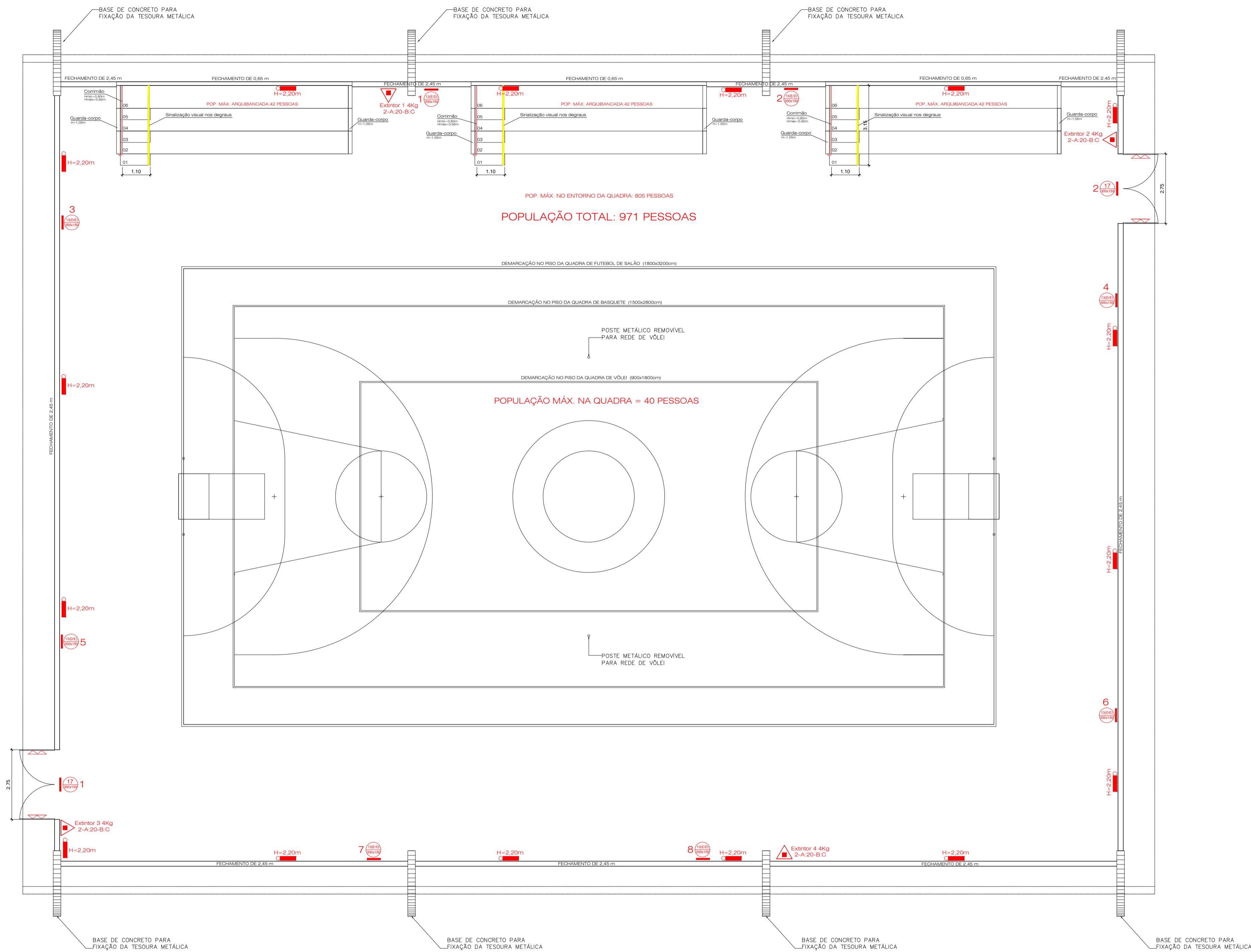
PLANTA BAIXA DO GINÁSIO POLIESPORTIVO ESCALA - 1:100
