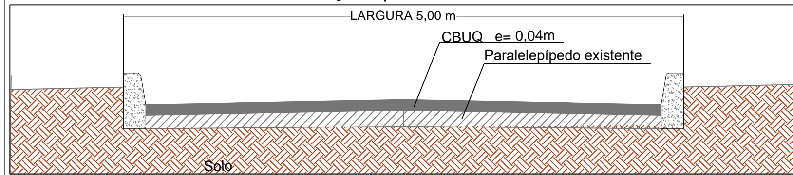
Seção Tipo
