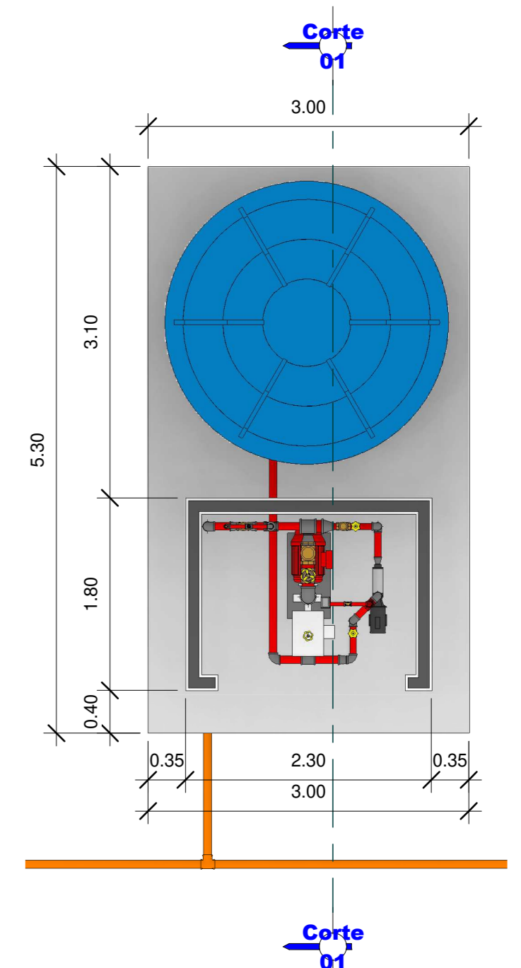
3 Detalhe Reservatório de casa de máquinas 1 : 50
