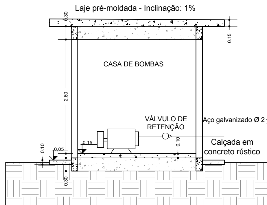
03 CORTE A A 1/50 A= 9,00 M 2
