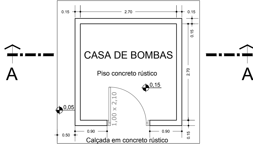
01 PLANTA BAIXA TÉC. 1/50 A= 9,00 M 2
