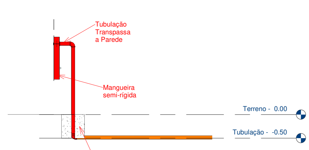
9 Detalhe 02 1 : 50
