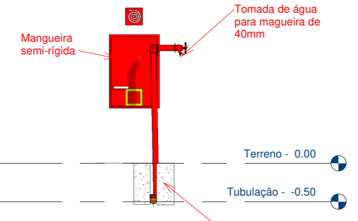
8 Detalhe 01 1 : 50
