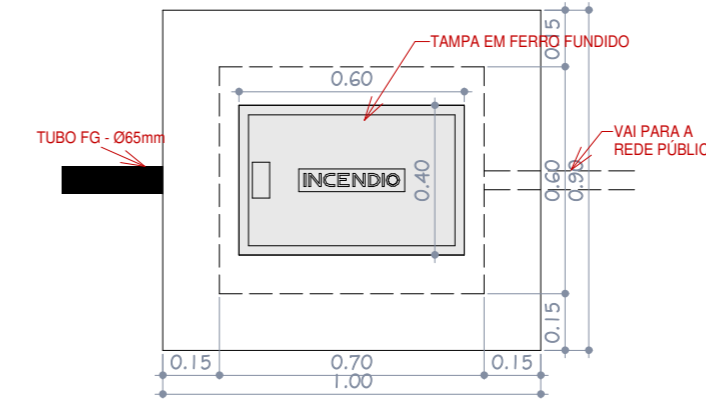
6 DET. HIDRANTE PASSEIO 1 : 20
