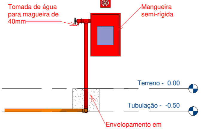
7 Detalhe 03 1 : 50
