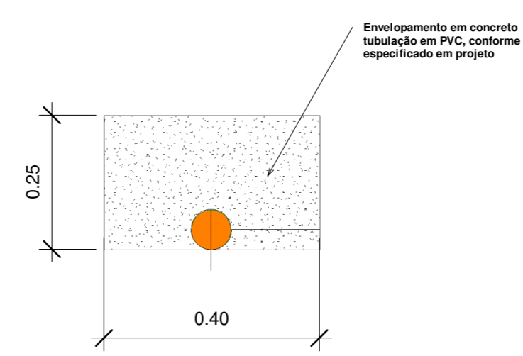
4 Detalhe Envolvimento em Concreto 1 : 10
